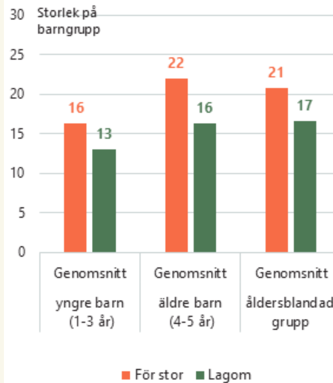
Diagram 3. Genomsnittlig gruppstorlek beroende på upplevelse om gruppstorleken
